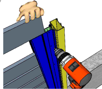
בניית משקוף עם השלבים בהברגה
