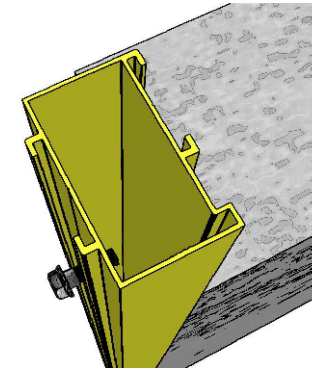
פילוס עמודי הגדר לחומה וחיבור ע"י בורג גמבו
